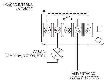
Figura 05 – Modelo de Ligação do Timer
