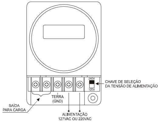
Figura 02 - Vistas frontal e conexões timer TM-6331
